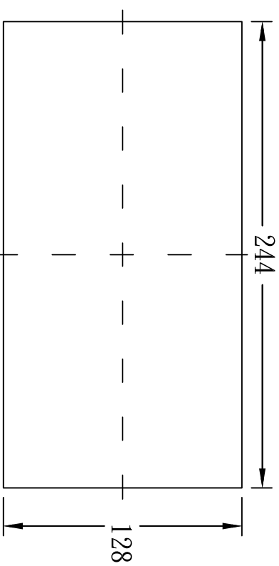
EPC 開孔圖
