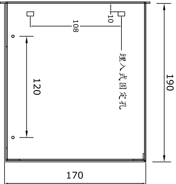
LPC控制器側邊
