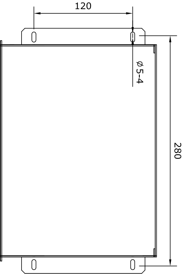
LPC控制器底部安裝
